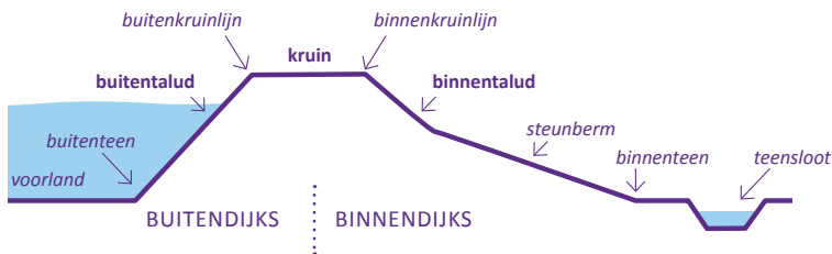
Schema dijkprofiel
